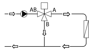
Valvola deviatrice utilizzata in deviazione
