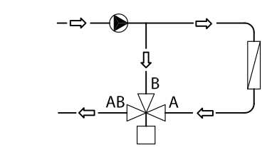
Valvola miscelatrice utilizzata in deviazione
